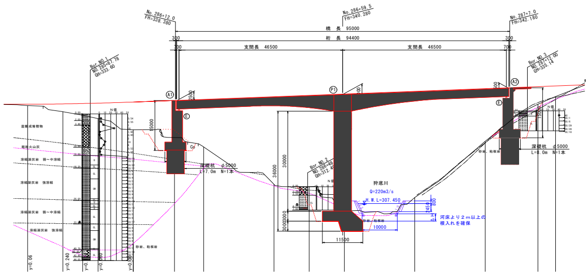
側面図
