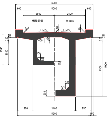
上部工標準断面図
